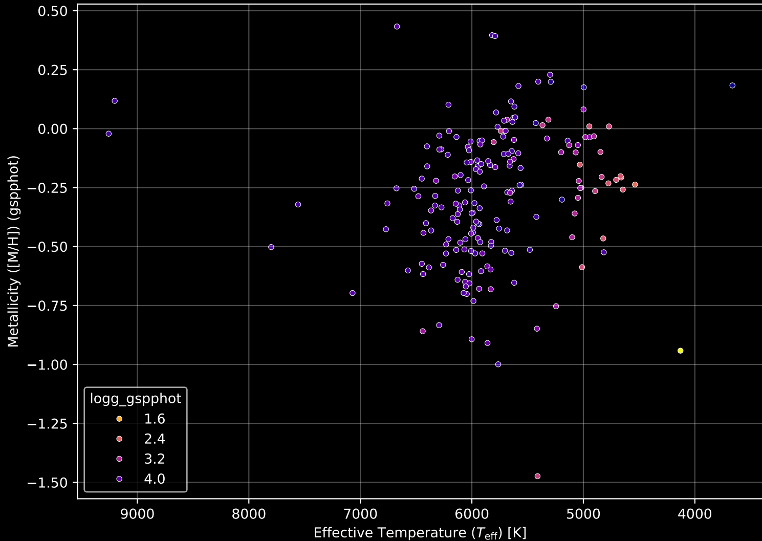
GALAH DR4 Field: [403] Stellar Population Parameters (n= 190)
