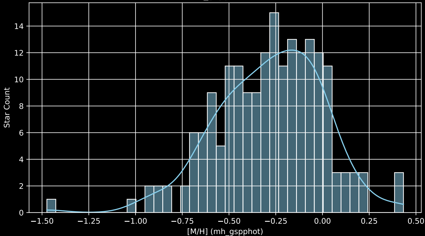
GALAH DR4 Field: [403] [M/H] (mh_gspphot) (n= 190)
