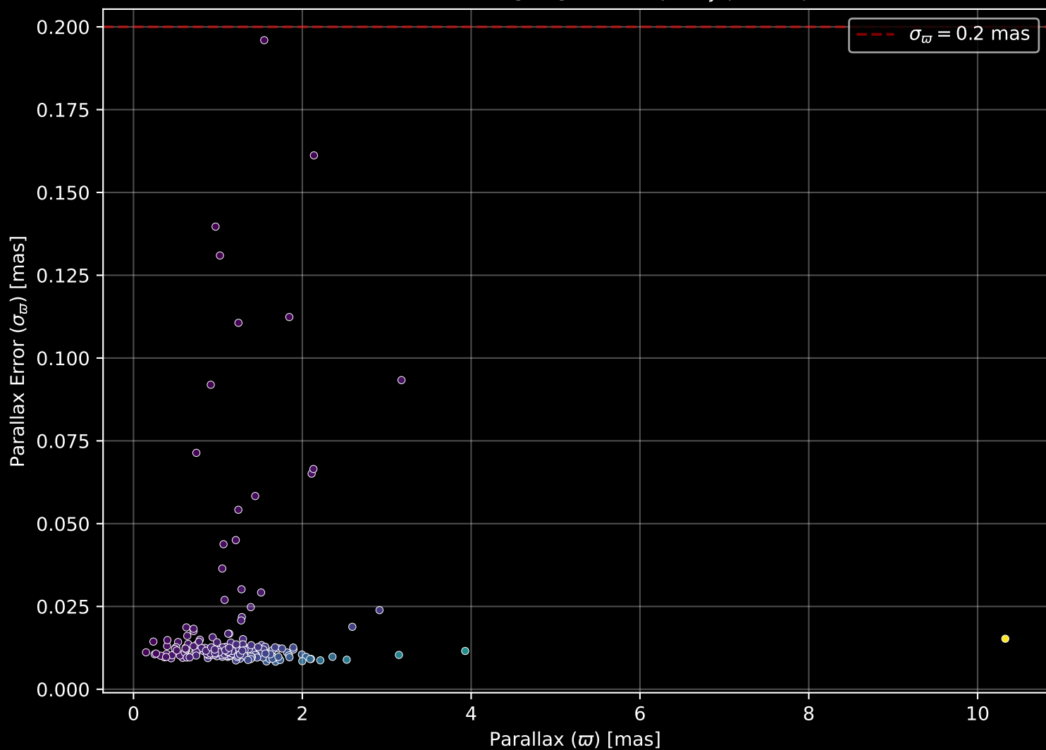
GALAH DR4 Field: [403] Parallax Quality (n= 190)
