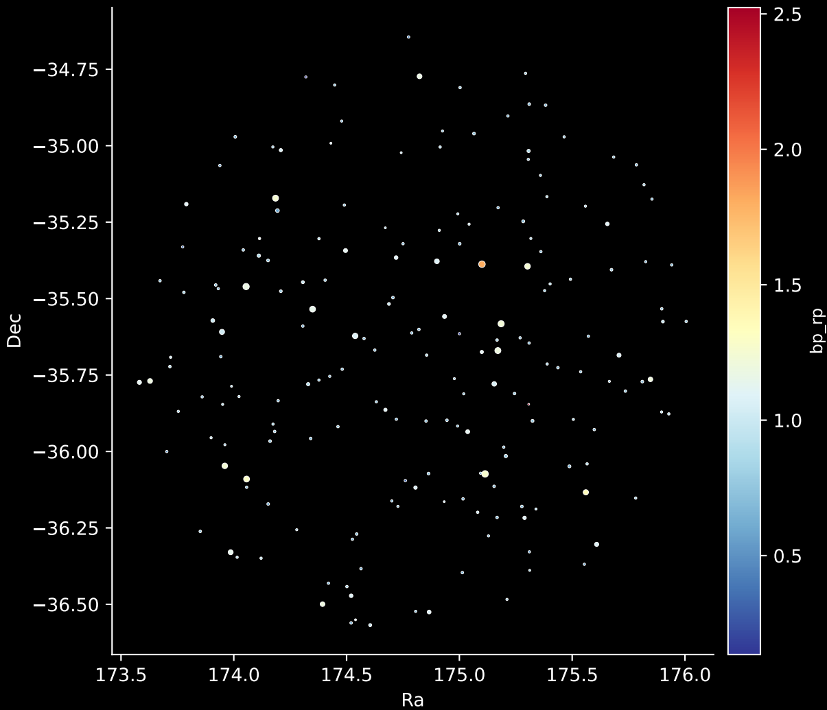
GALAH DR4 Field: [403] Stars: 190
